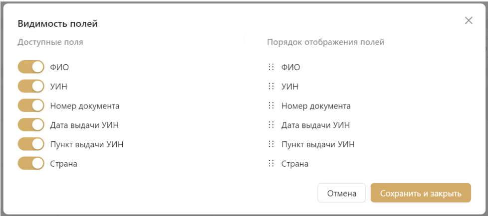
Рисунок 3.2.3 – Настройка столбцов
