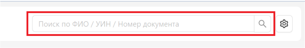
Рисунок 3.2.1 – Поиск
