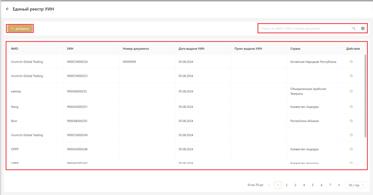
Рисунок 3.1 – Функционал
