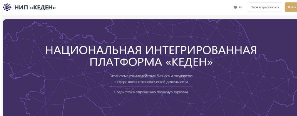
Рисунок 1 – Авторизация
