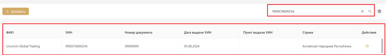
Рисунок 3.2.2 – Результат поиска
