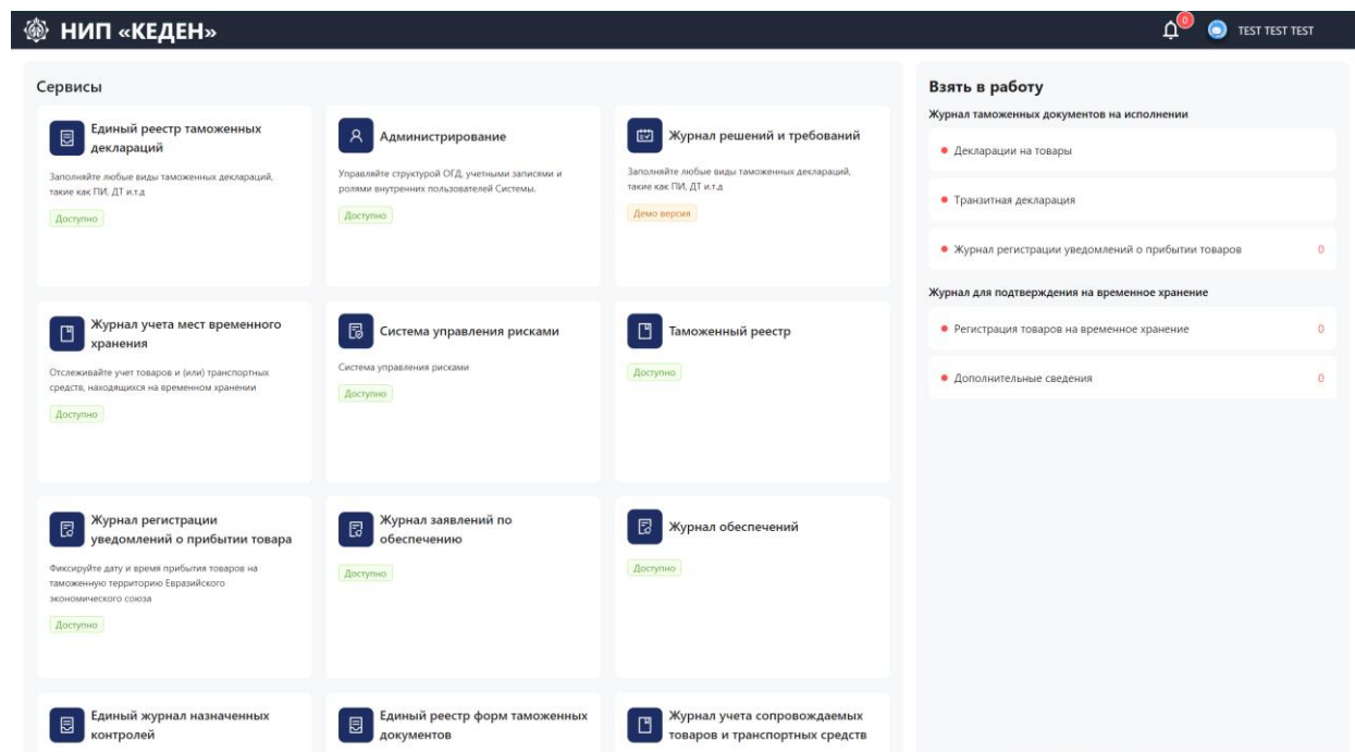
Рисунок 2 – Главная страница
